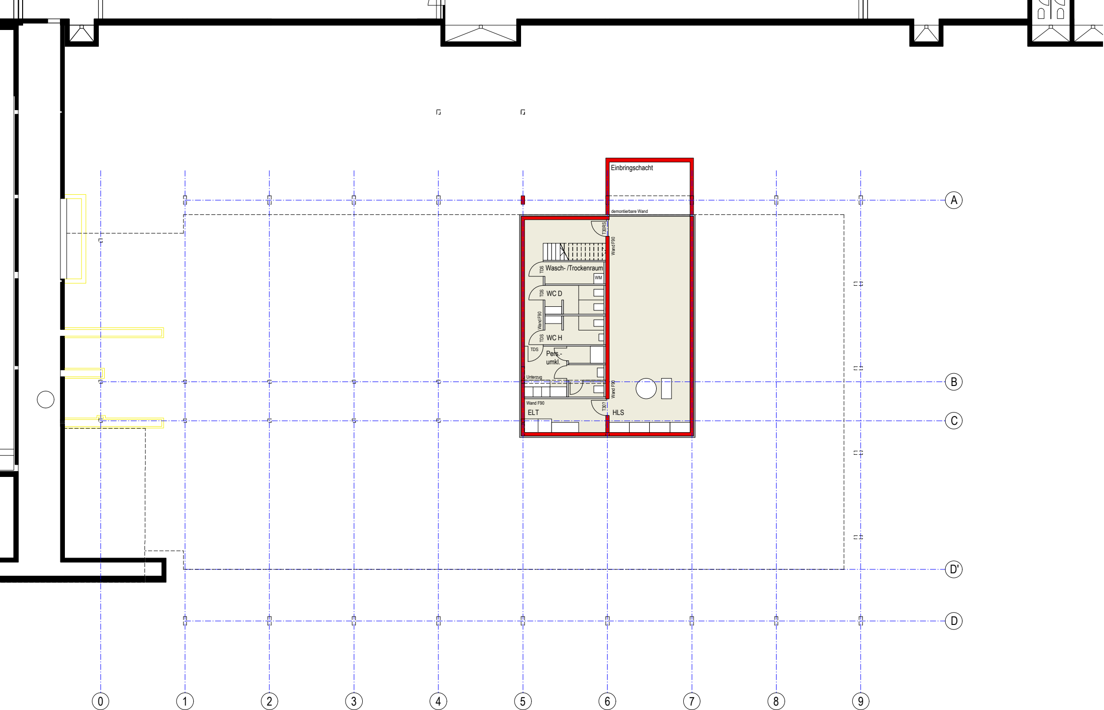
Schlösslesfeldschule Erweiterung Ganztagesbetreuung, Mensa / Entwurf / Grundriss Kellergeschoss
