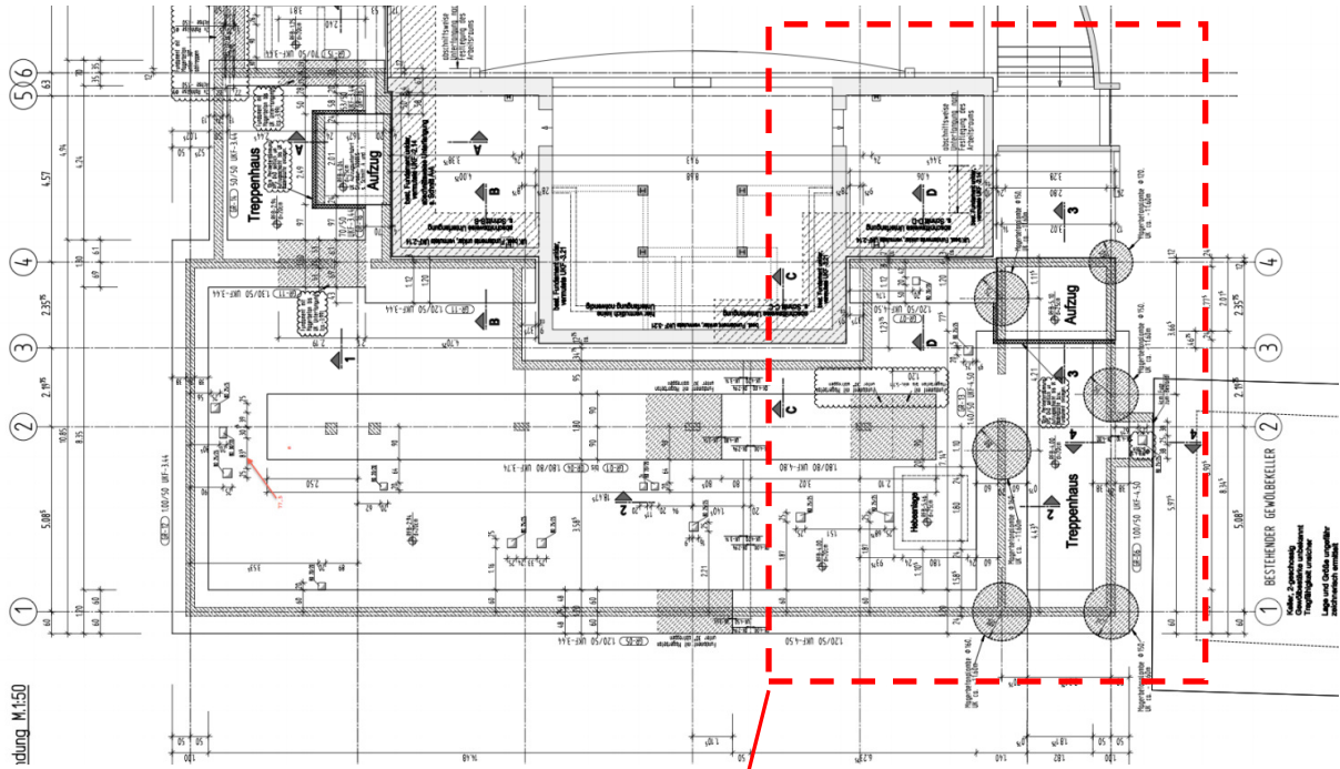
Plan Ausschnitt Gründung Neubau (Variante 1)
