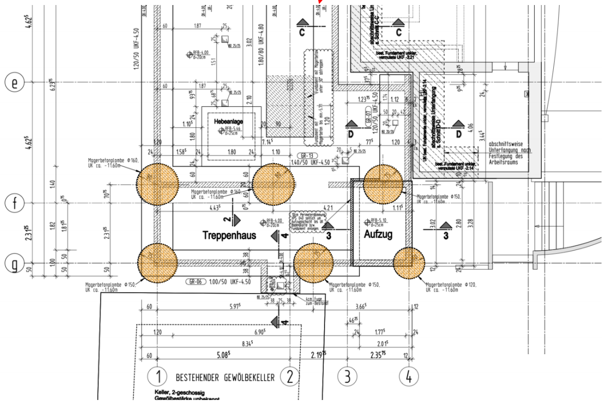
Notwendigkeit von Magerbetonplomben als Tiefgründung Plan Ausschnitt (ohne Maßstab)
