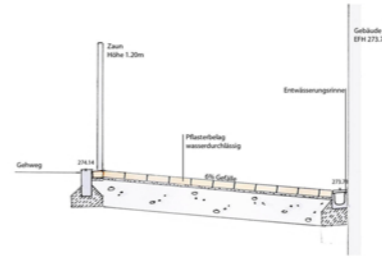
Schnitt B-B' M 1:50
