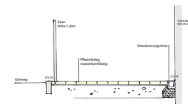
Schnitt C-C' M1:50
