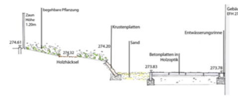
Schnitt A-A' M 1:50
