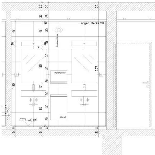
Wandansichten geplante Wasch- und Duschräume
