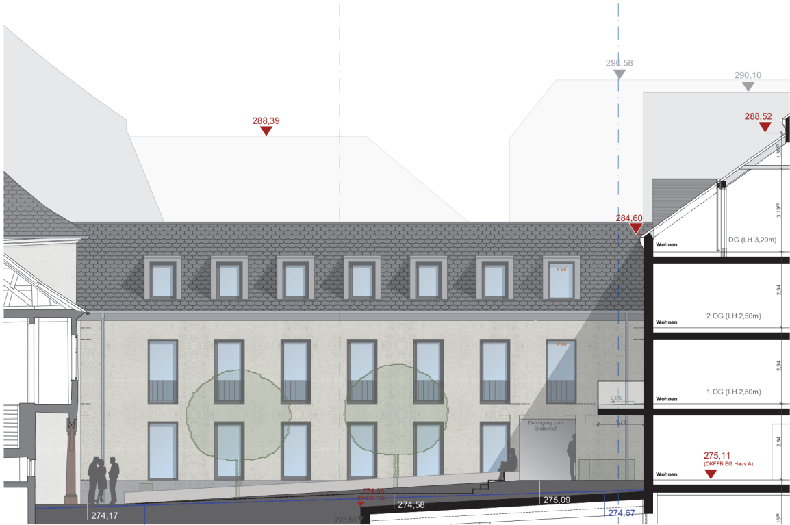
Nordansicht Haus F2 (F-F)
