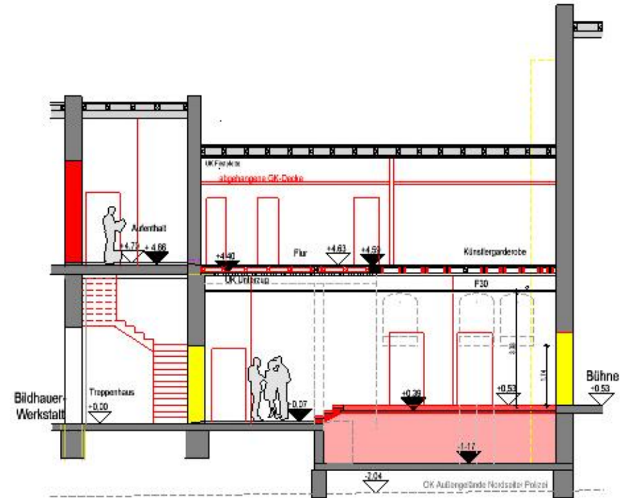
Schnitt C-C
