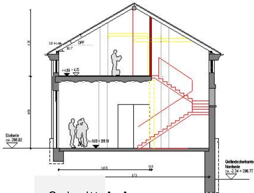
Schnitt A-A
