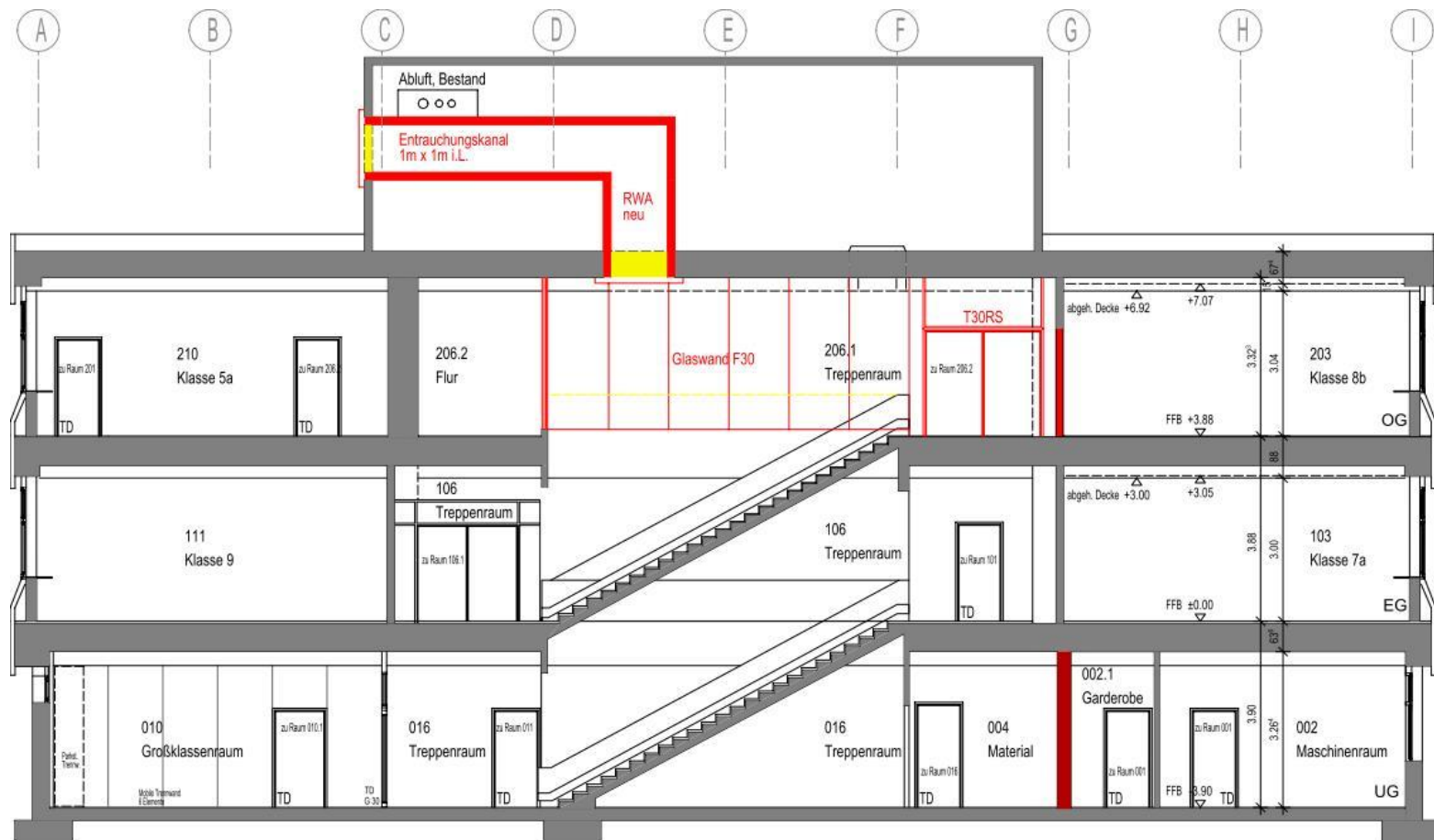
Schnitt 1-1
