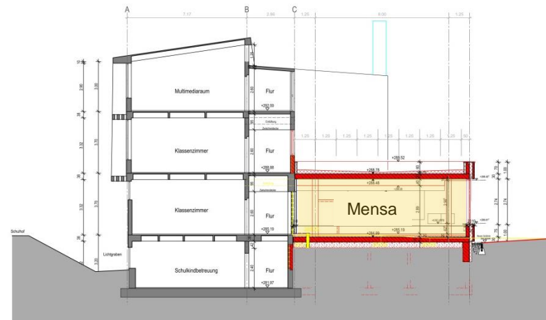
Schnitt 2
