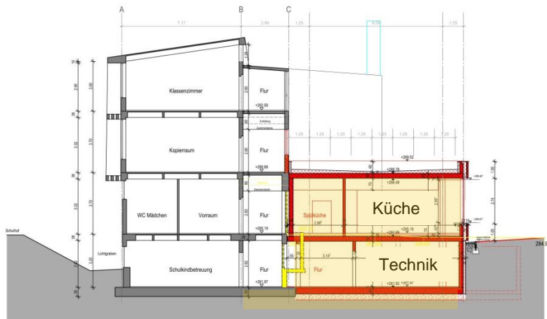
Schnitt 1
