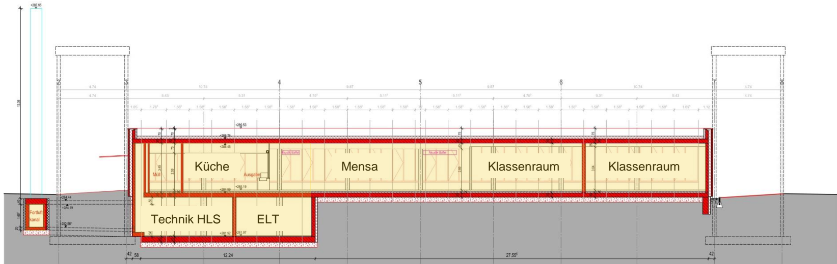
Längsschnitt
