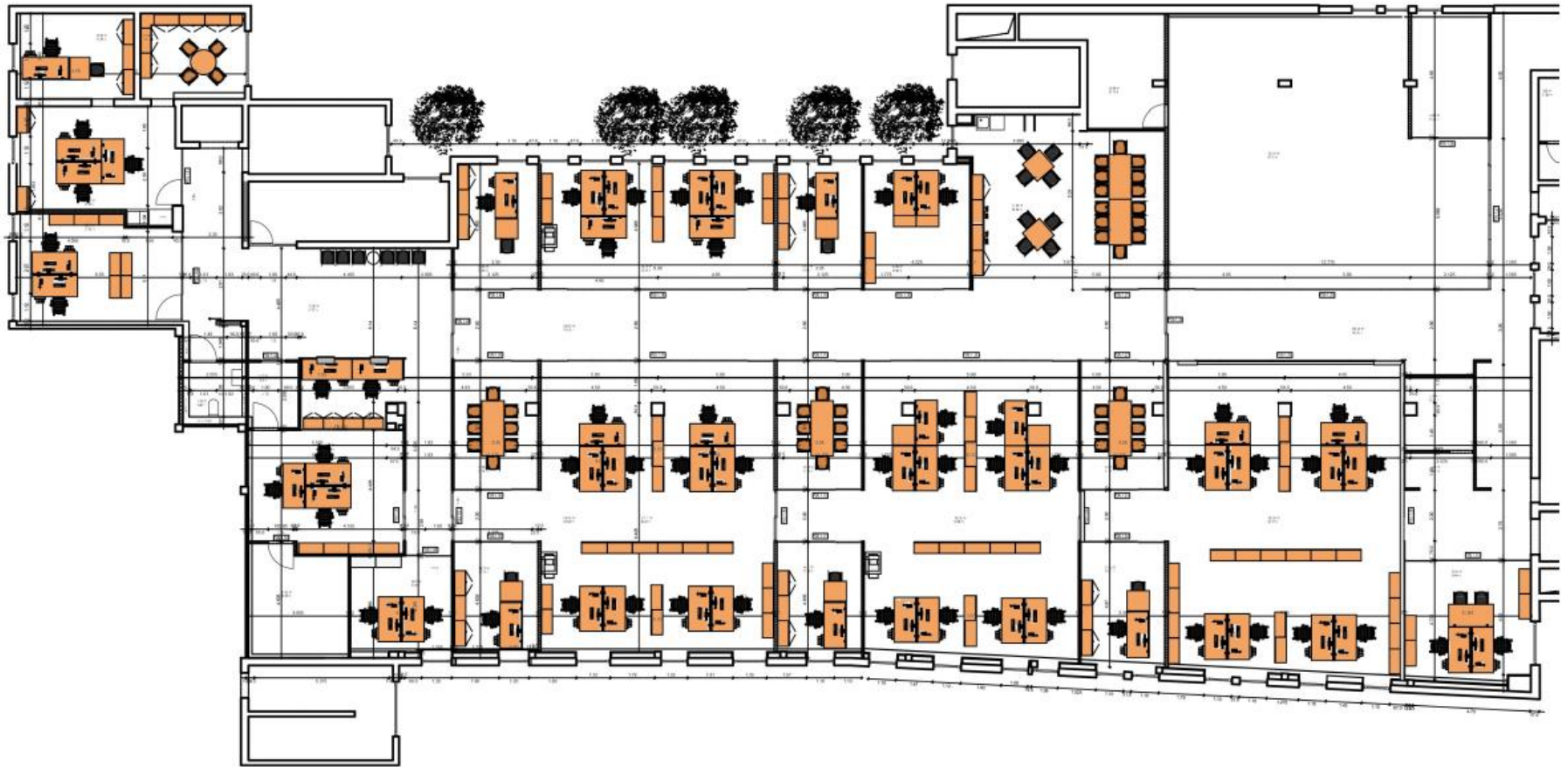
Grundriss mit loser Möblierung
