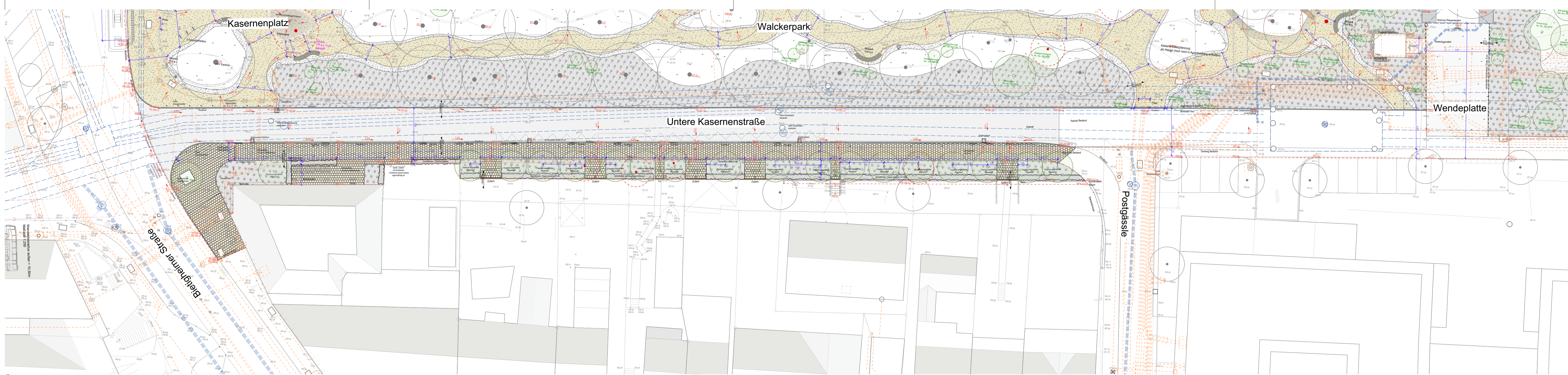
Übersicht Untere Kasernenstraße M 1: 250
