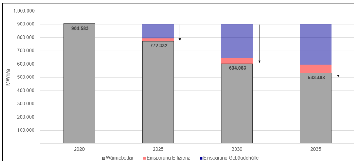
Abbildung 9: Energiebedarfsentwicklung – Szenario 1
