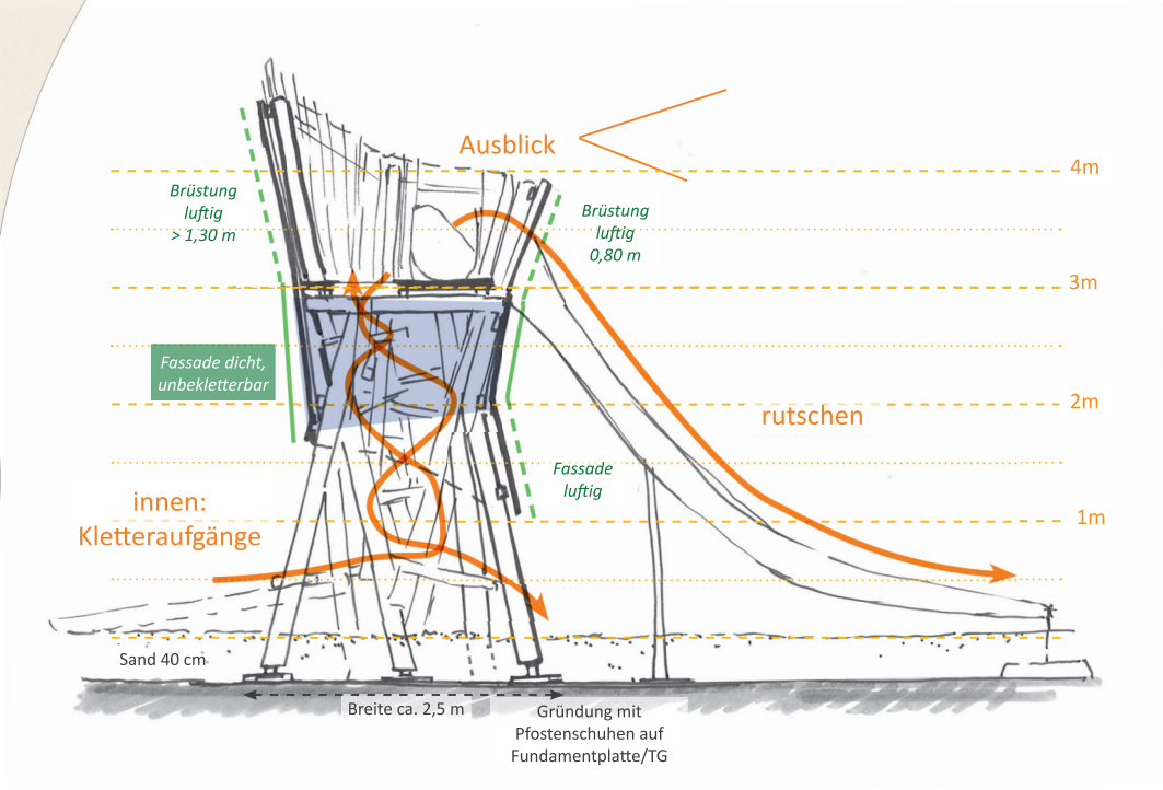
Schnittskizze
